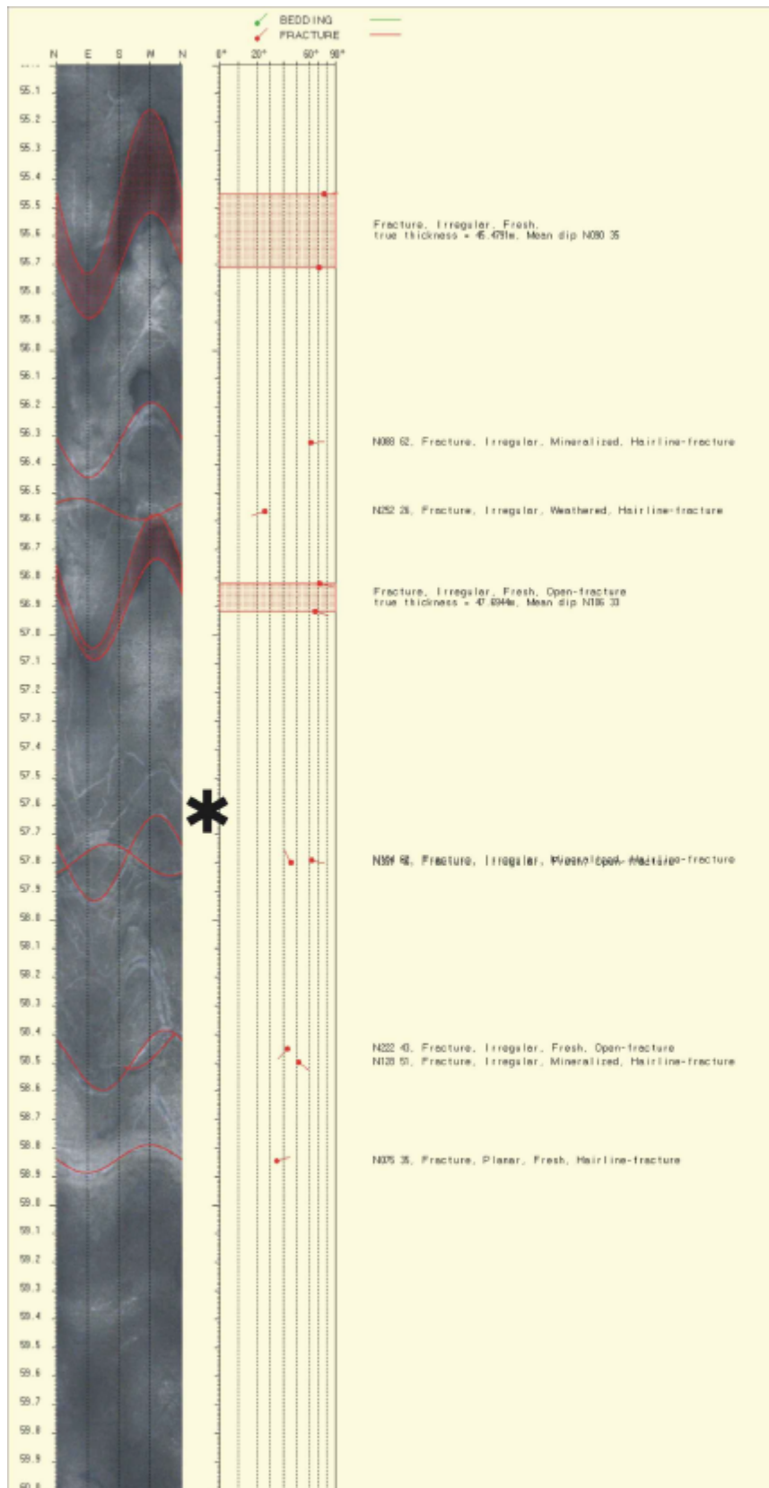
Figur 29: Bilde-logg borhull 8, 55-60 lpm.
