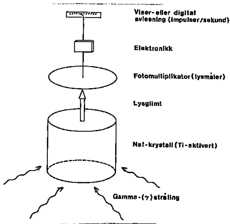
Fig. 4. Prinsippskisse for oppbygging av scintillometer eller scintillasjonsteller
