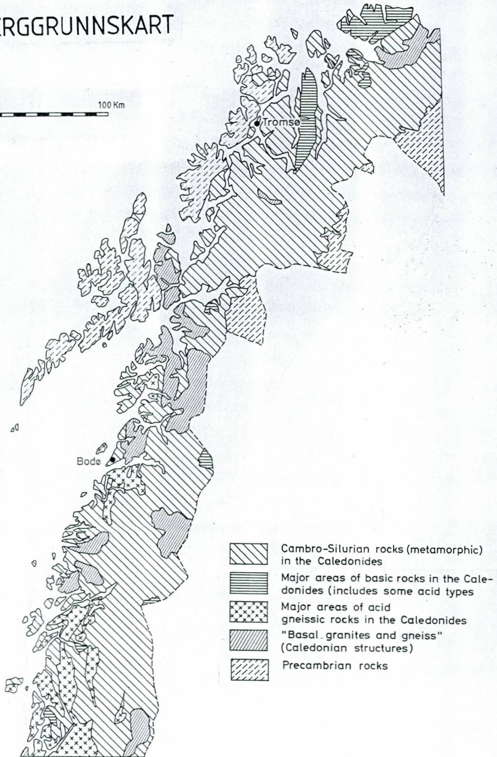
Figur 2. Geologisk oversiktskart
