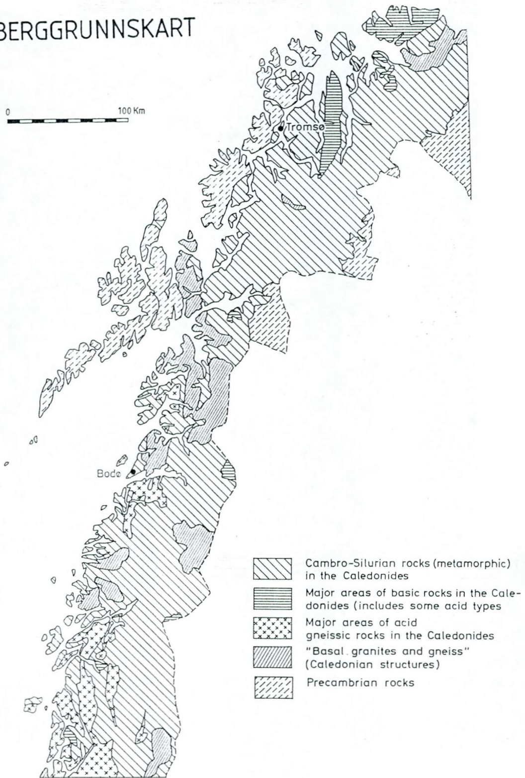
Figur 2 Geologisk oversiktskart
