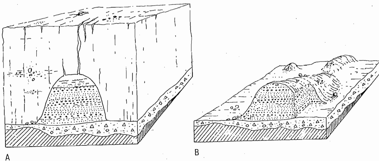
Fig. 8: DANNEELSE AV ESKER
