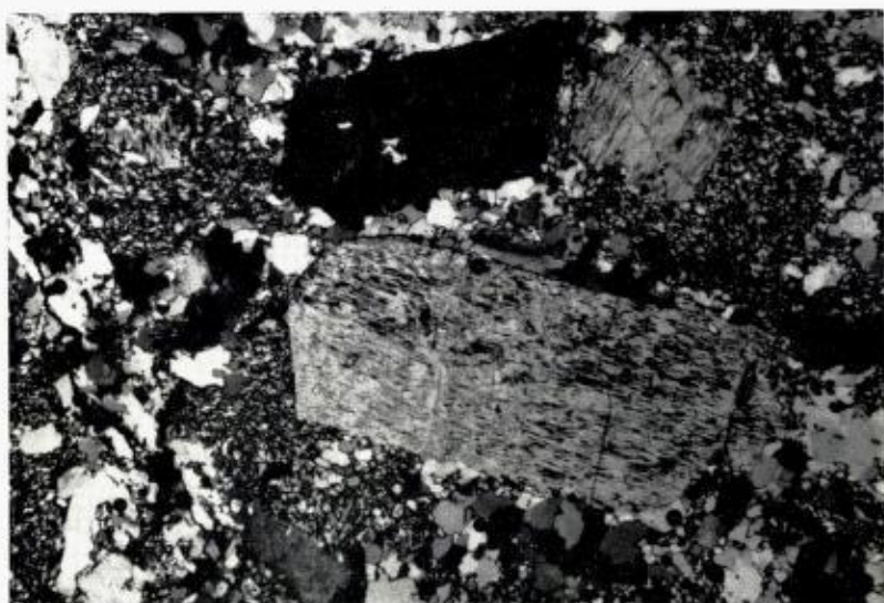
Foto 6. Blastofyrisk tekstur i kvartskeratofyr der den primære feltspat er omvandlet til sjakkbrettalbite. x31. Blastopphyric texture in quartzkeratophyre. The primary feldspar is altered to chess- board albite. x31.
