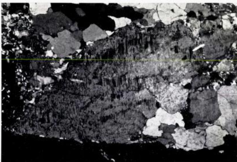
Foto 10. Sjakkbrettalbite med årer som i grov åreperthitt og sannsynligvis et omdannelsesprodukt av åreperthitt. Fra den nordlige del av den sentrale granittsone. x44. Chessboard albite, veined as in coarse vein perthite and probably an alteration of this mineral. From the northern part of the central granite zone. x44.
