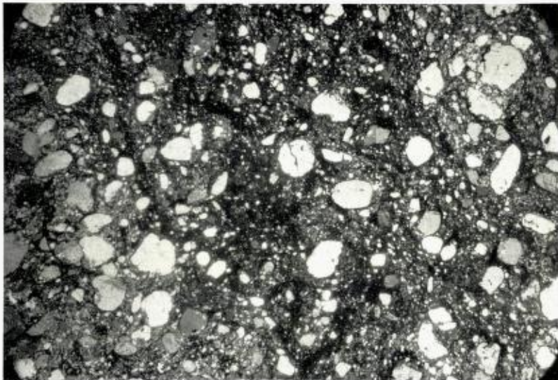
Foto 7. Rundede plagioklaskorn i en kloritrik matrix. Fra en metagråvakkevariant. x7. Rounded plagioclase grains in a chlorite-rich matrix. From a variant of the metagraywacke. x7.
