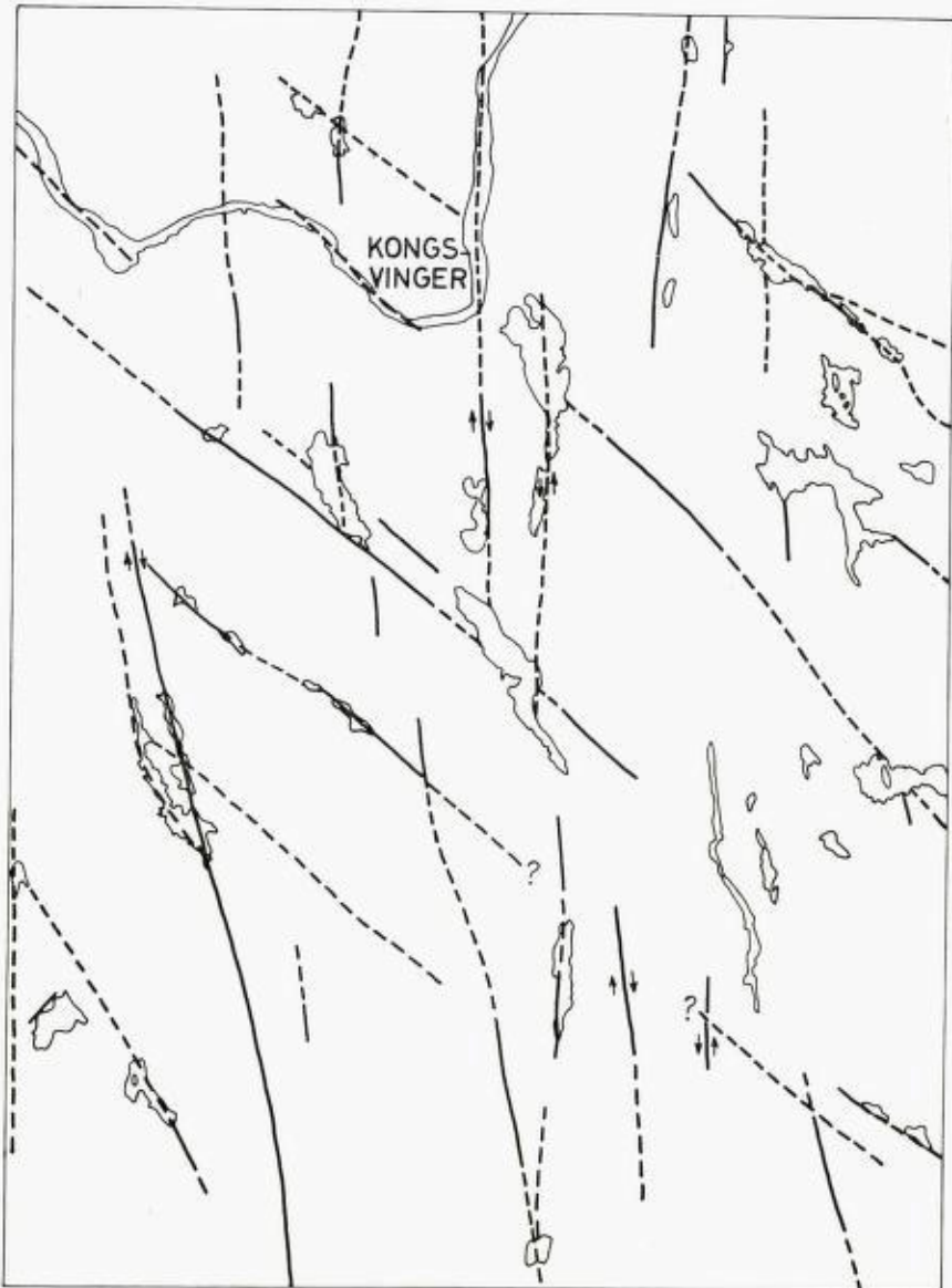
Fig. 3. Breksjesoner på kartblad Kongsvinger. Hel strek — observert breksje, stiplet strek — antatt breksje etter terrengformasjonene. Breccia zones on the map AMS Kongsvinger. Full line — observed breccia, broken line — probable breccia.
