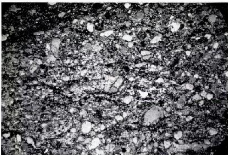
Foto 8. Mulig klastisk tekstur i metagråvakke med kantede og delvis rundede plagioklaskorn. x7. Possible clastic texture in metagraywacke with angular and partly rounded grains of plagioclase. x7.
