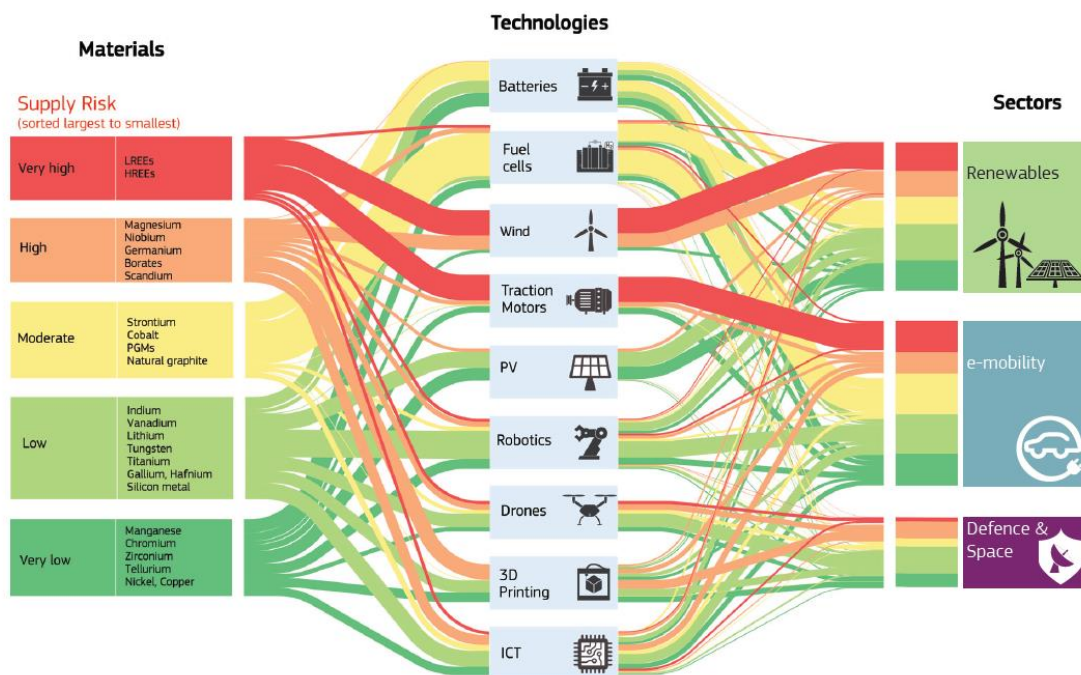
Figur 3: Illustrasjon som viser (fra venstre mot høyre) metallene gruppert etter forsyningsrisiko, deres bruksområder og sektorer i samfunnet (Bobba et al. 2020).
