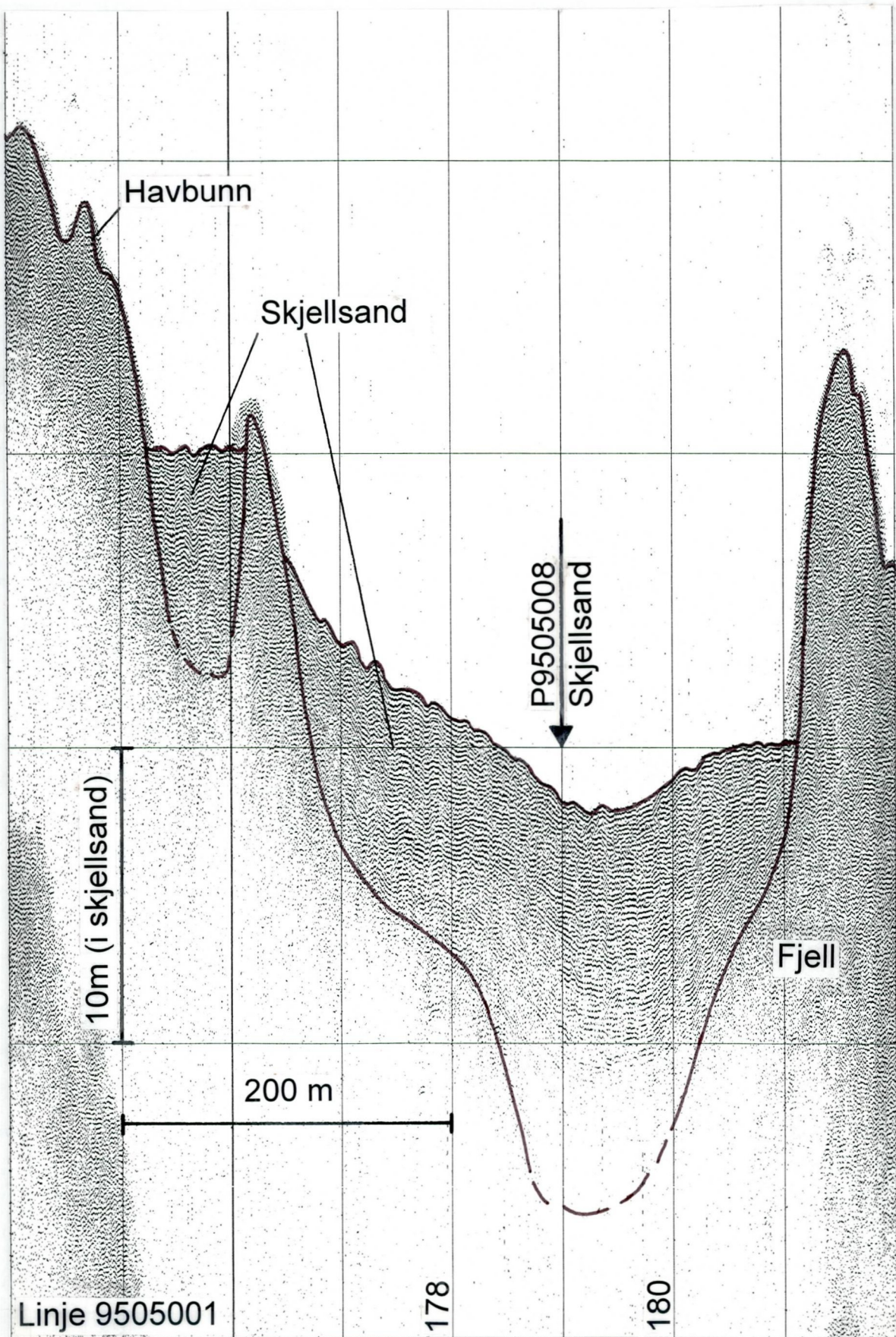
Fig. 1. Eksempel på tolket refleksjonsseismisk profil fra Bømlo.
